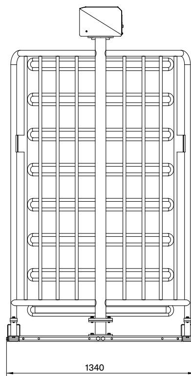
MPT *3* vormontiert – Ansicht von der Seite
