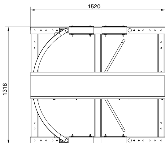
MPT *3* vormontiert – Ansicht von oben
