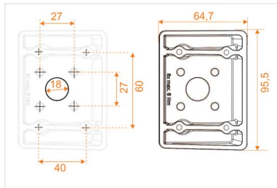
Abmessungen Montagekeil 30°
