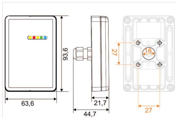
Abmessungen Radar-Scanner
