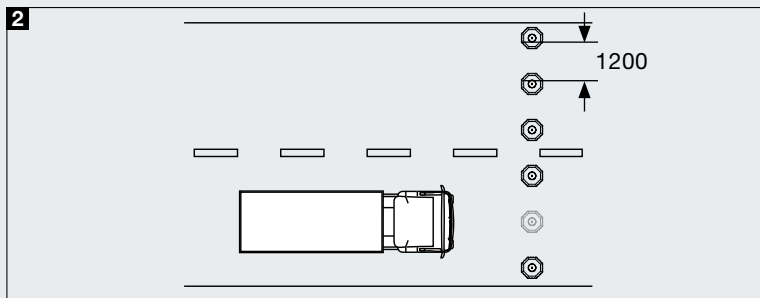
Absperrung in unbegrenzter Breite mit der Möglichkeit, schnell und einfach Durchlassmöglichkeiten für berechnigte Fahrzeuge zu schaffen
