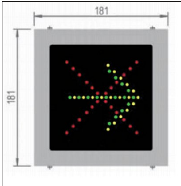
im Gehäuse für Innenbereiche (Außenmaße 181 x 181 mm)
