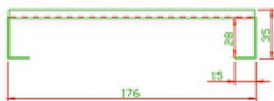
Lochblech für OEM Einbau (Maße 176 x 176 mm, 35 mm tief)
